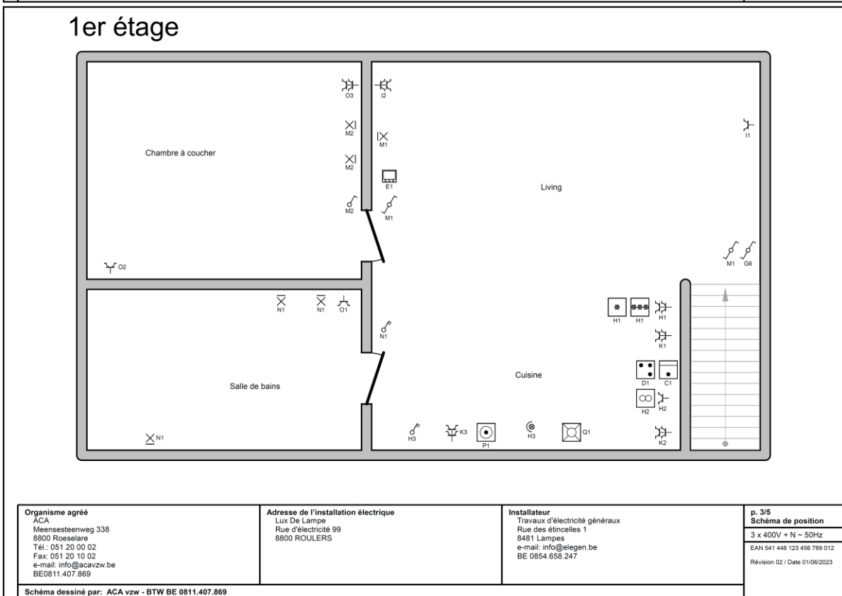
Figure 14 – Exemple d'un plan de position
