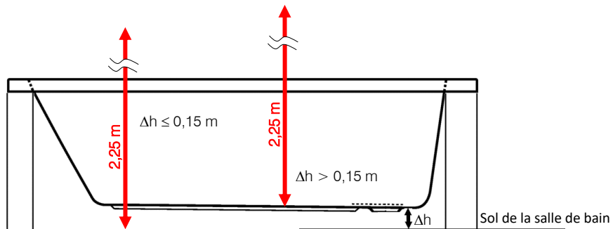
Figure 12 – Détermination de la hauteur du plan horizontal supérieur
